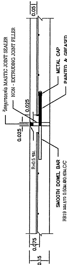
ขมบรอยต่อ EXPANSION JOINT
